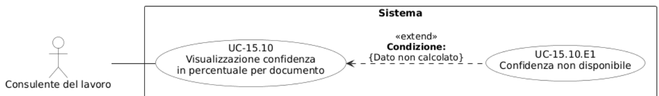
Figura 63: Diagramma del caso d'uso UC-15.10: Visualizzazione confidenza in percentuale per documento
